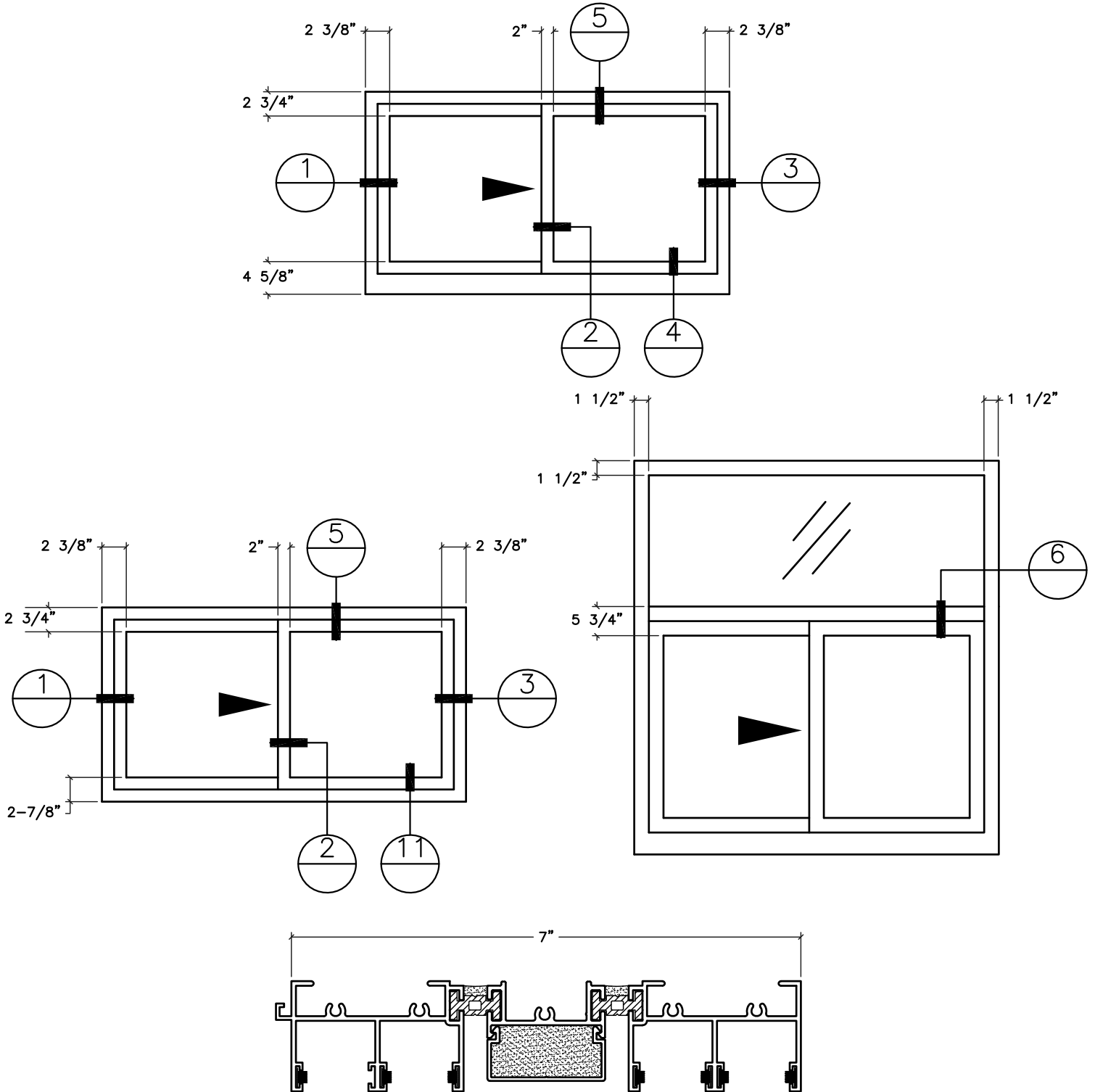
A7 ACOUSTIC FRAME
