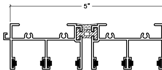
900 STD. FRAME
