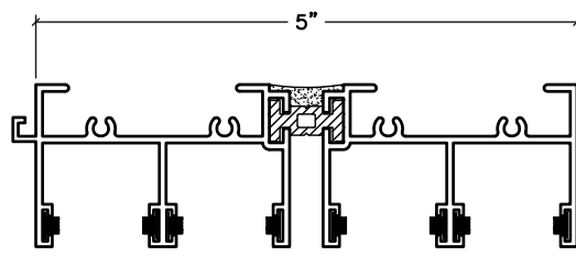
900 STD. FRAME
