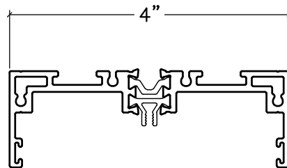
4000 STD. FRAME
