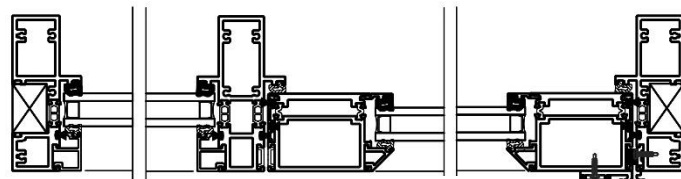
4500 ENTRANCE DOOR
