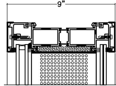
9000 CURTAIN WALL
