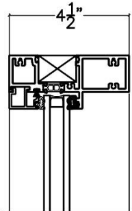
4500 STOREFRONT
