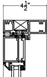
4500 ENTRANCE DOOR
